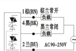
N图 交流三线制常开+常闭
