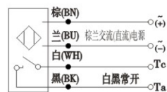
R图 四线制继电器触点输出
