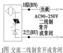
J图 交流二线制常开或常闭
