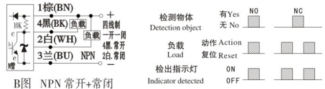
B图 NPN 常开+常闭
