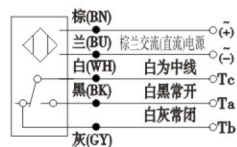
K图 五线制继电器触点输出
