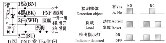
D图 PNP 常开+常闭
