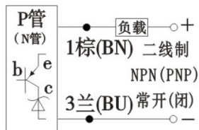
E图 PNP(NPN) 常开或常闭
